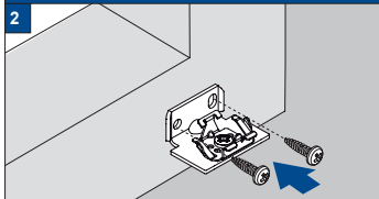
De afdekkappen boven aanbrengen
