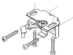
Spannriegel für Rollo aus Holz und Raffrollo aus Holz
